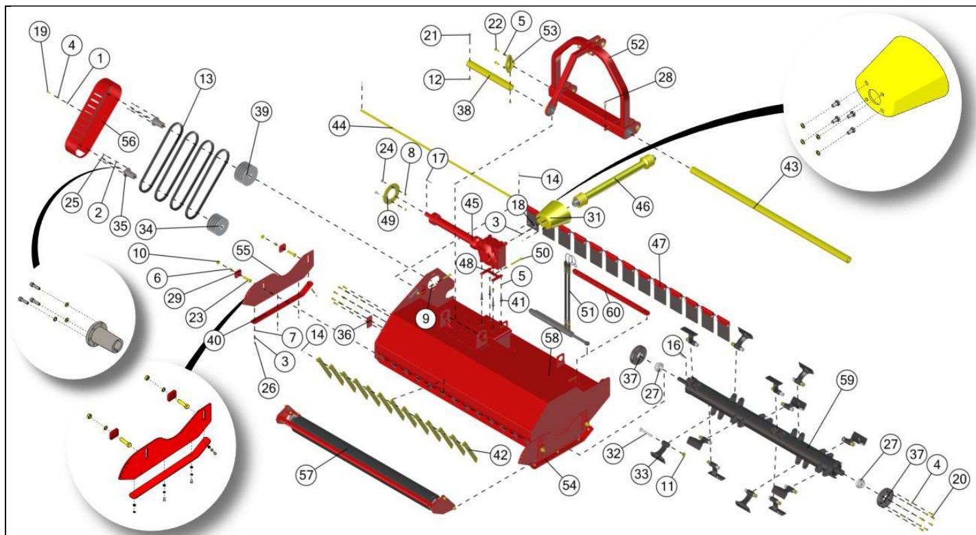
TRITURADOR TCP
