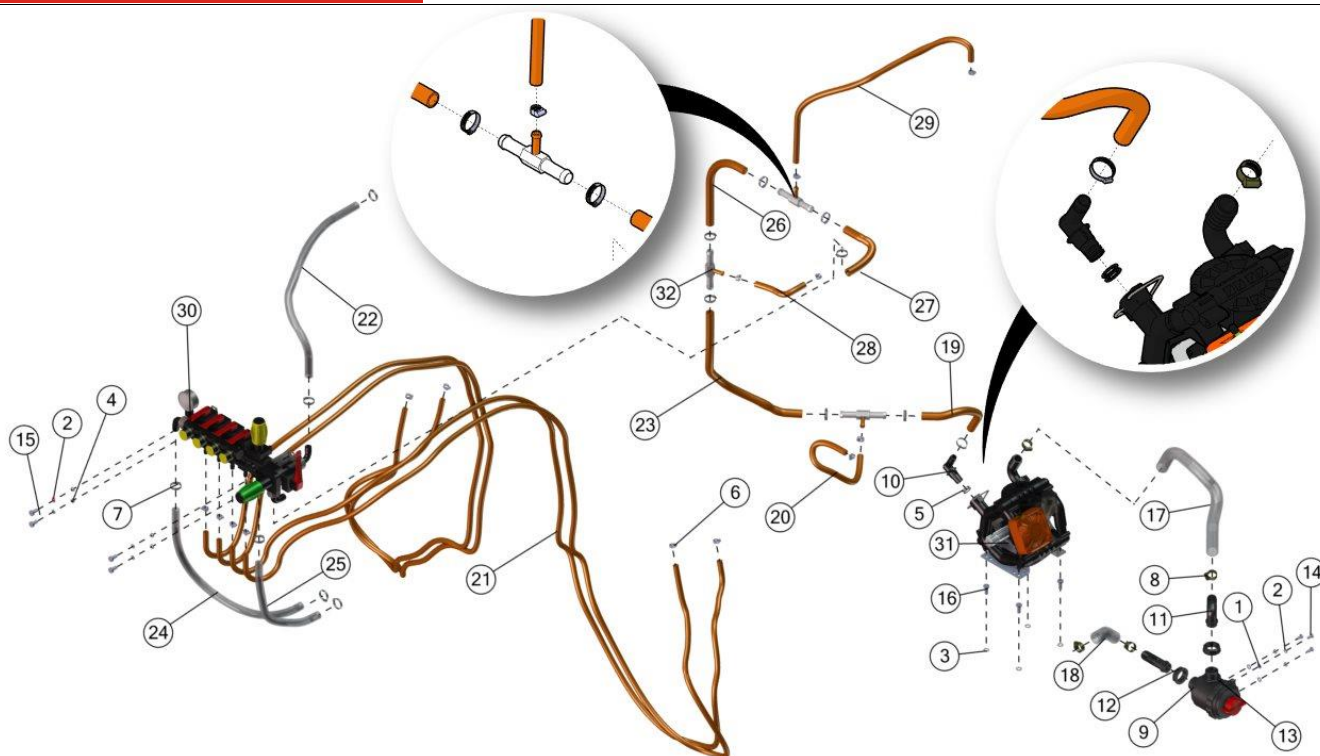
CIRCUITO HIDRÁULICO – 4 VIAS
