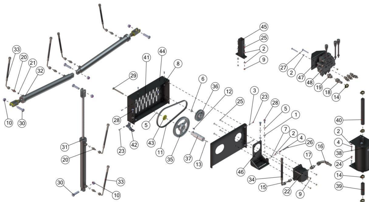
KIT CIRCUITO HIDRÁULICO DA BARRA
