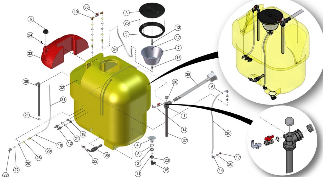
RESERVATÓRIO – 600 e 800 LITROS
