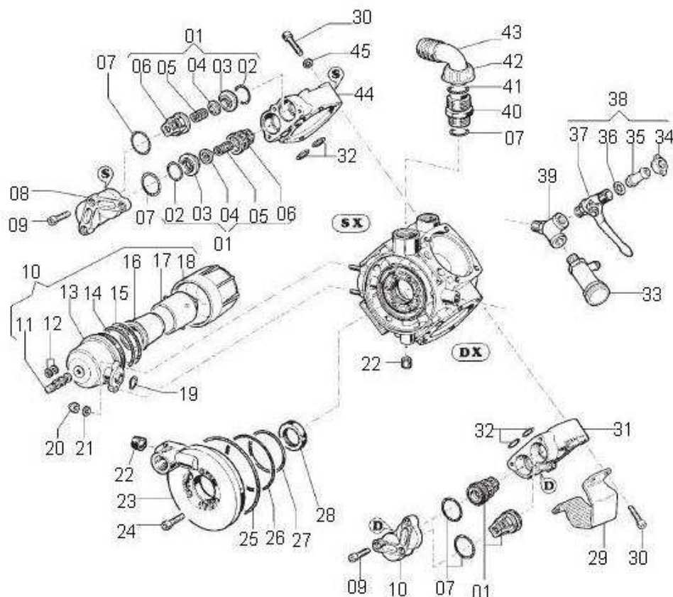
BOMBA APS-96
