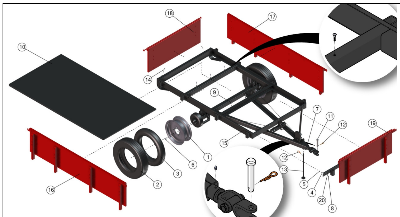
CARRETA AGRÍCOLA / CB-3
