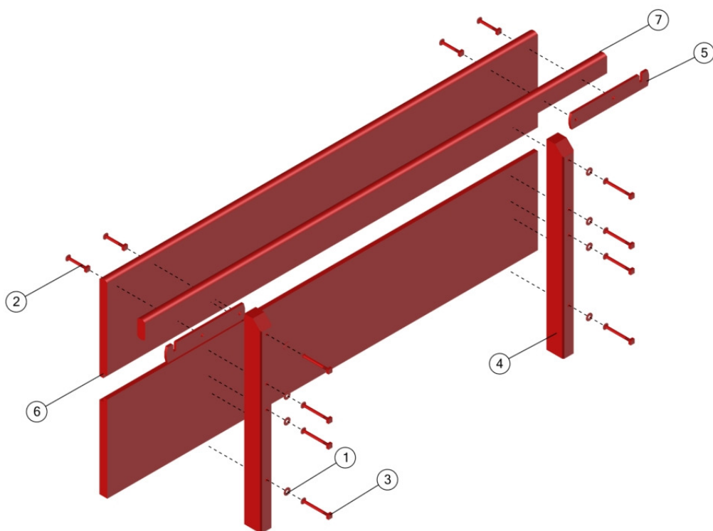
TAMPA DIANTEIRA – CB-3
