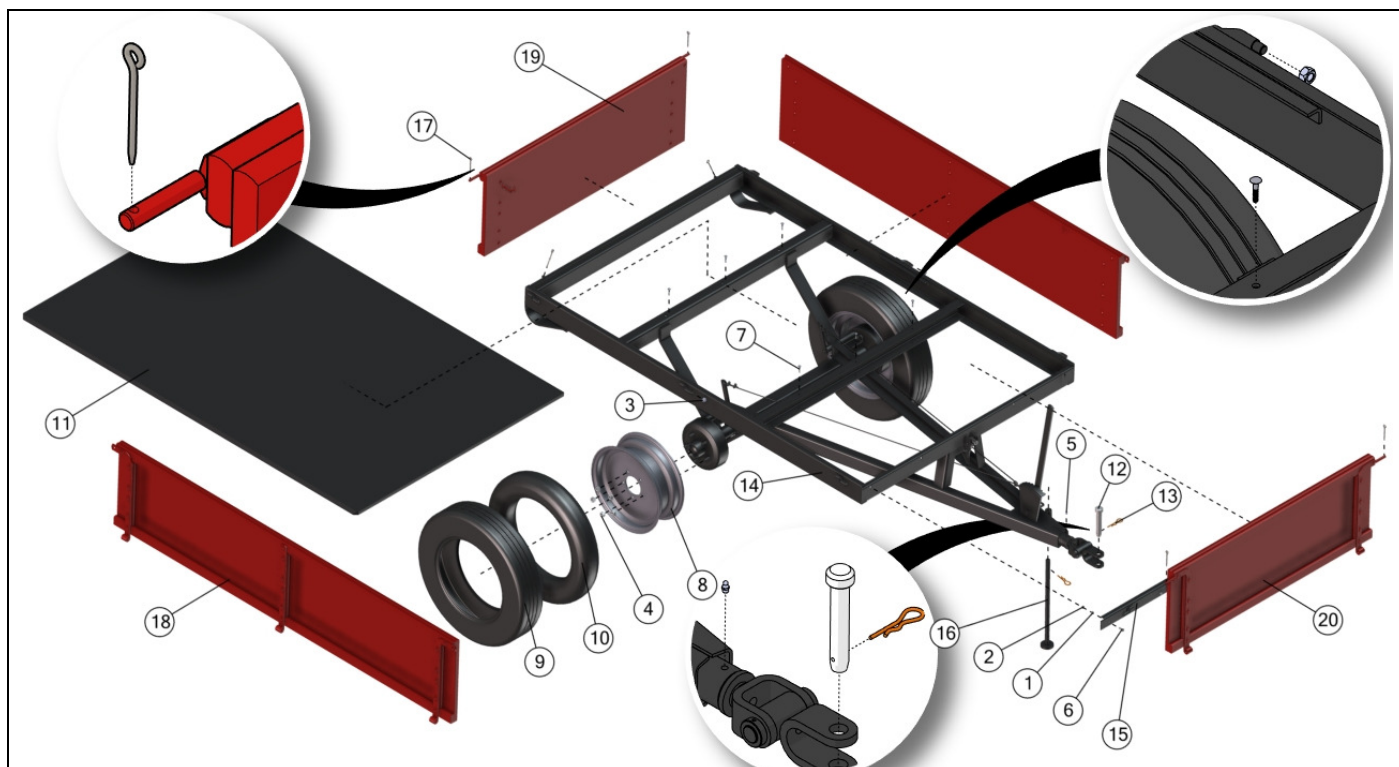
CARRETA AGRÍCOLA / CB-2
