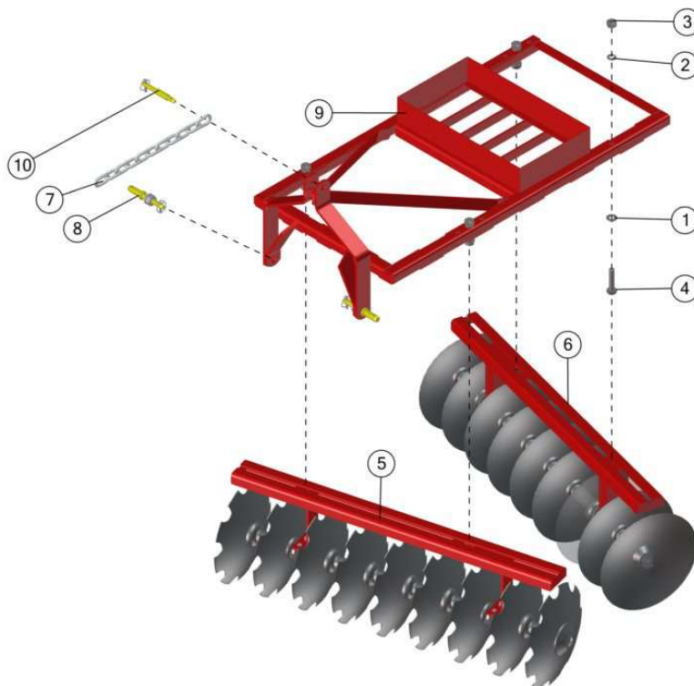
GRADE DE DISCOS – GVV 18x18"
