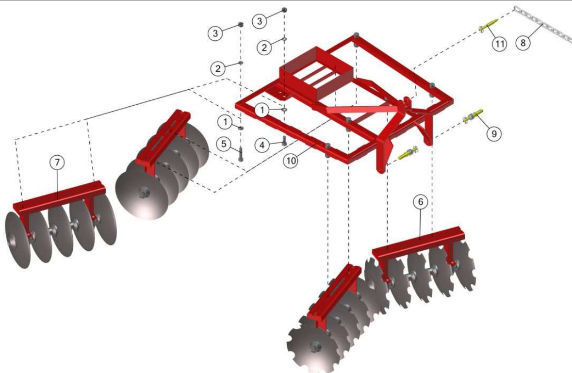
GRADE DE DISCOS – GXU 20x18"
